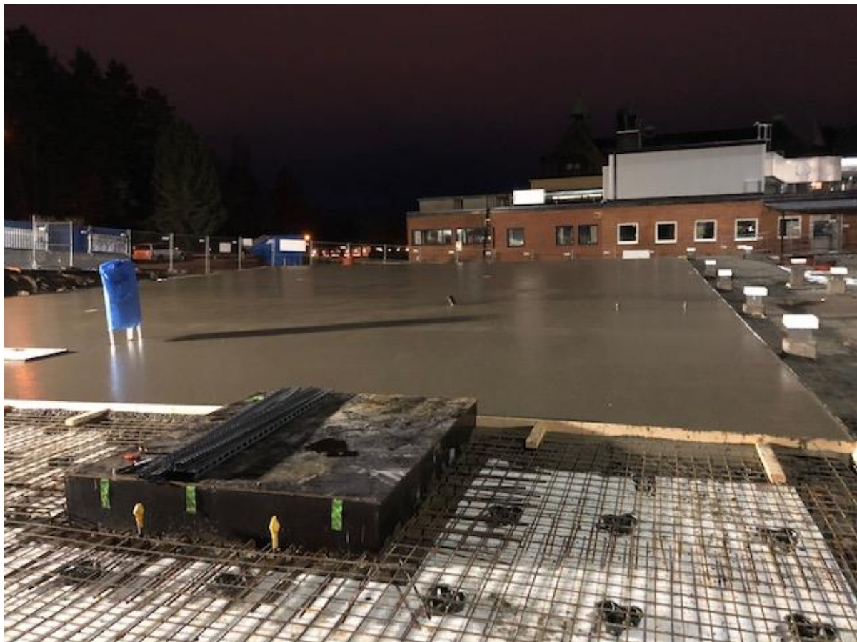
Drygt 70 m 3 senare. Hus 4 bottenplatta.
