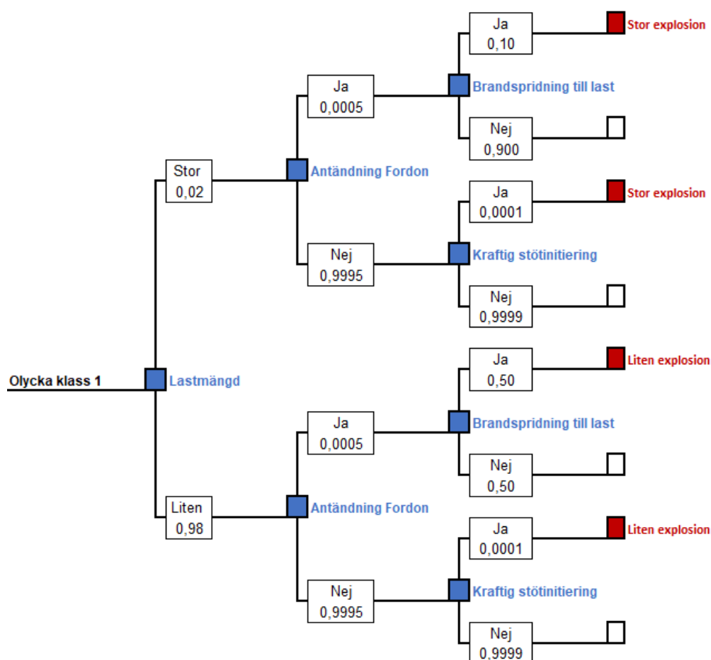
Figur 3-1. Händelseträäd för olycka med explosiva ämnen och föremål.
