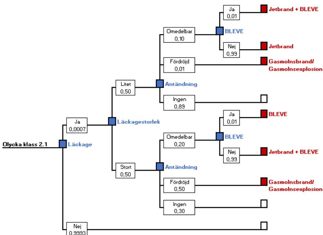
Figur 3-2. Händelseträd för olycka med brandfarlig gas.
