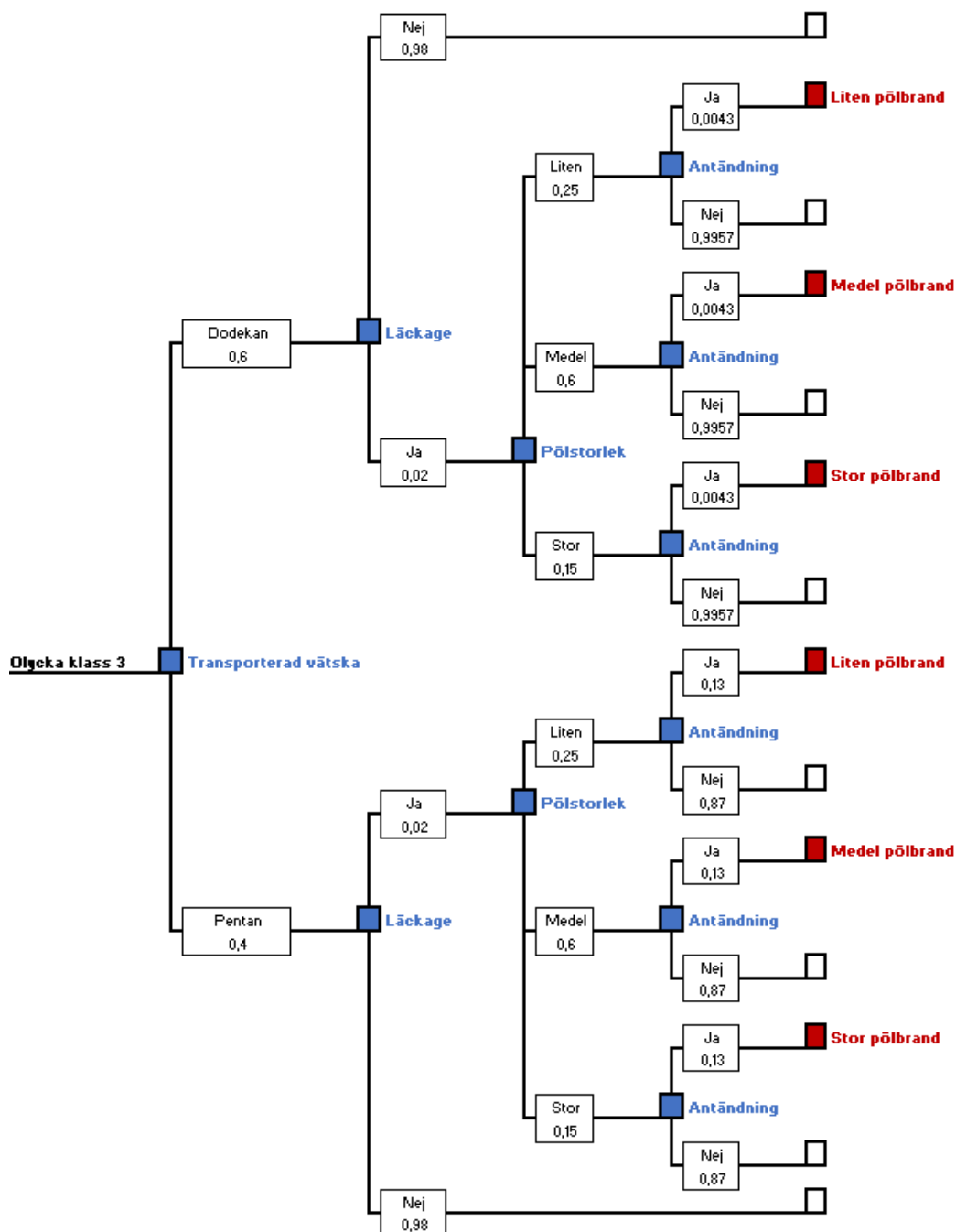
Figur 3-5. Händelseträd för olycka med brandfarlig vätska.
